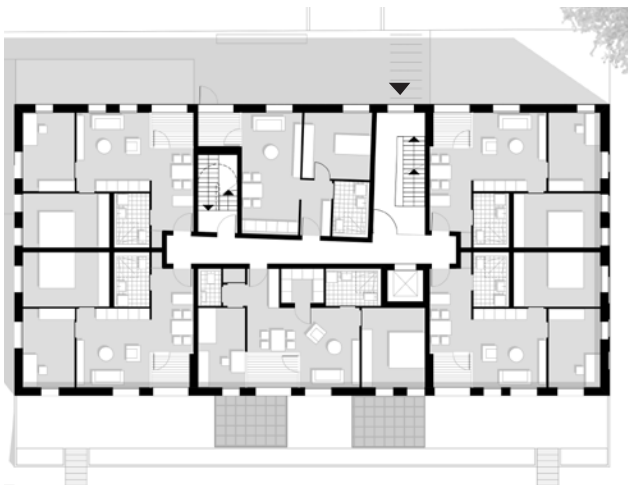
Grundriss EG
