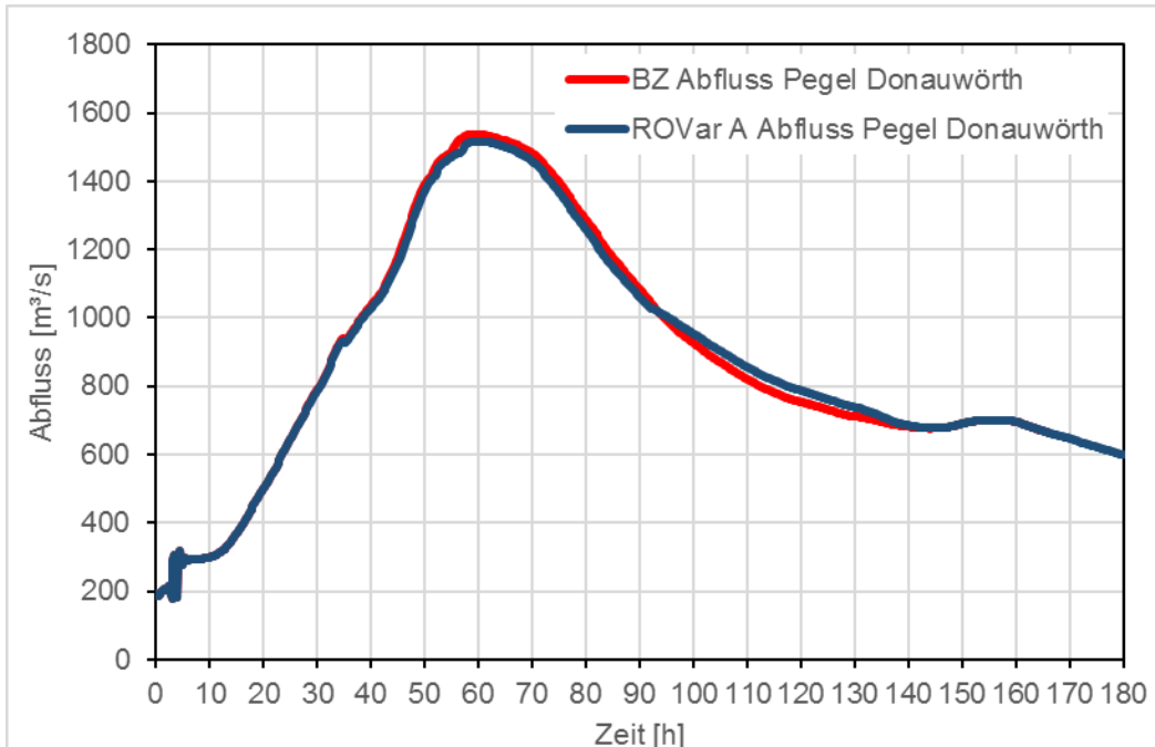
Abbildung 42: Pegel DON, ROVar A - Projektteilziel 3, Abflussganglinien
