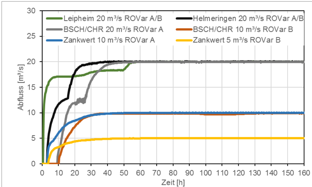
Abbildung 61: Ökologische Flutungen Abfluss am Auslass, Füllvorgang
