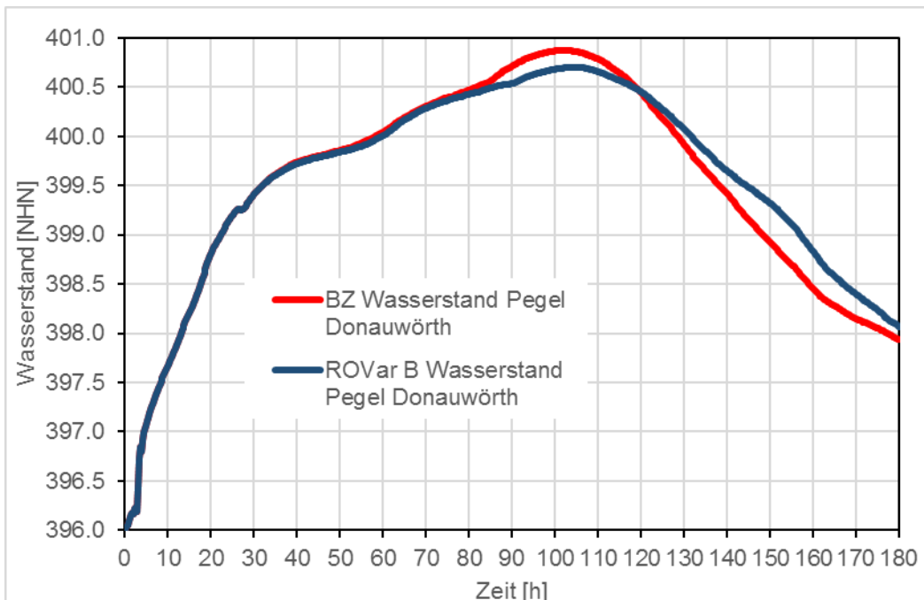
Abbildung 54: Pegel DON, ROVar B - Projektteilziel 1, Pegelganglinien
