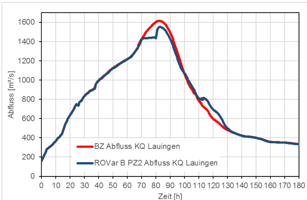
Abbildung 47: Helmeringen ROVar B - Projektteilziel 1, Abflussganglinien Kontrollquerschnitt Lauingen
