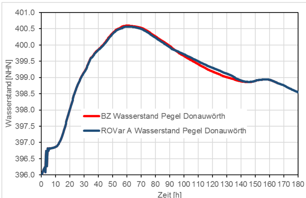
Abbildung 43: Pegel DON, ROVar A - Projektteilziel 3, Pegelganglinien
