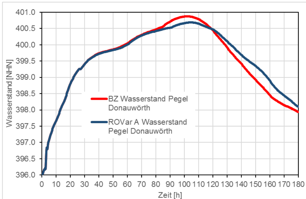
Abbildung 40: Pegel DON, ROVar A - Projektteilziel 1, Pegelganglinien
