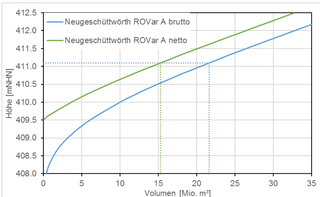
Abbildung 14: Speicherinhaltslinie Rückhalteraum Neugeschüttwörth ROVar A
