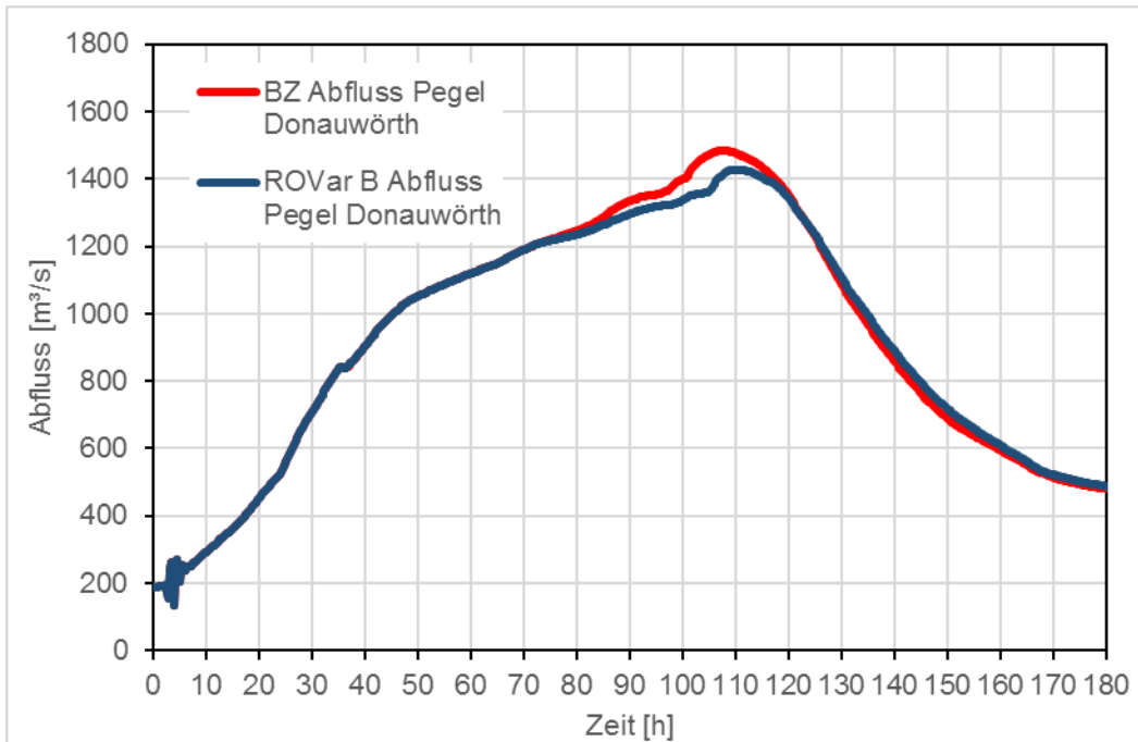
Abbildung 59: Pegel DON, ROVar B - Projektteilziel 2, Abflussganglinien
