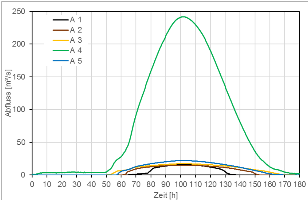
Abbildung 51: Neugeschüttwörth ROVar B - Projektteilziel 1, Abflussaufteilung Abflussbauwerke
