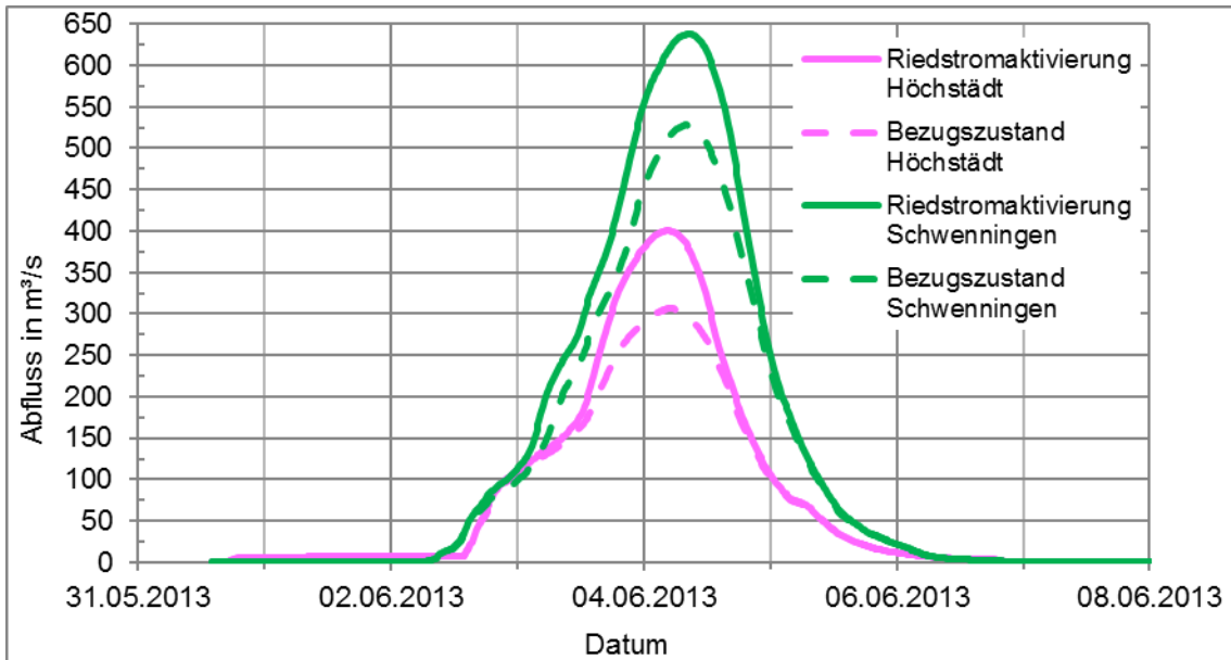
Abbildung 67: Abfluss im Riedstrom im Bezugzustand und im Fall der Riedstromaktivierung
