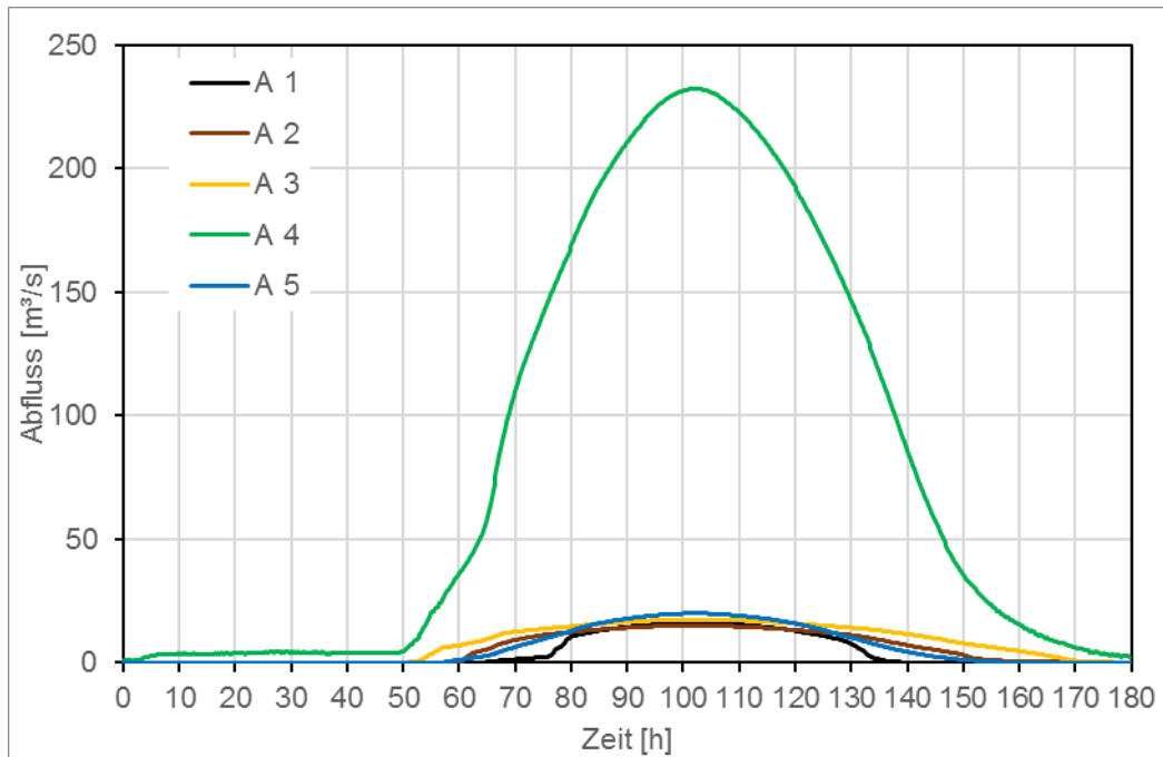
Abbildung 37: Neugeschüttwörth ROVar A - Projektteilziel 1, Abflussaufteilung Durchlassbauwerke
