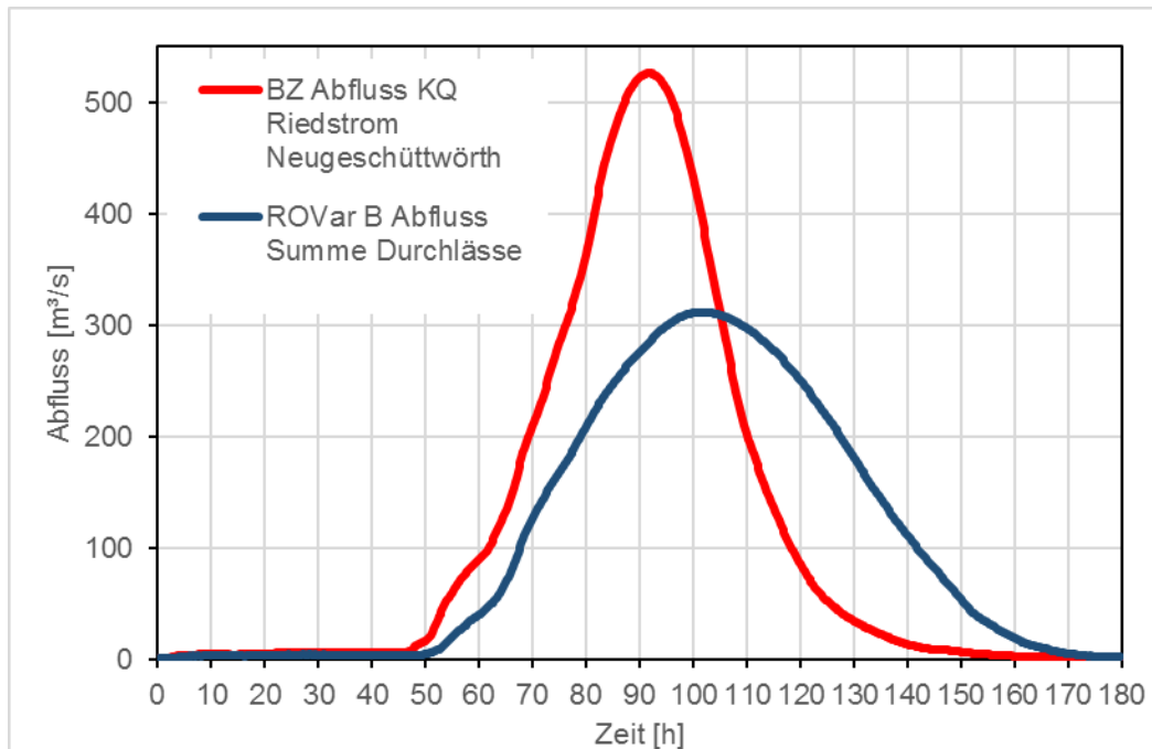
Abbildung 50: Neugeschüttwörth ROVar B - Projektteilziel 1, Ganглиe Kontrollquerschnitt bzw. Auslassbauwerke
