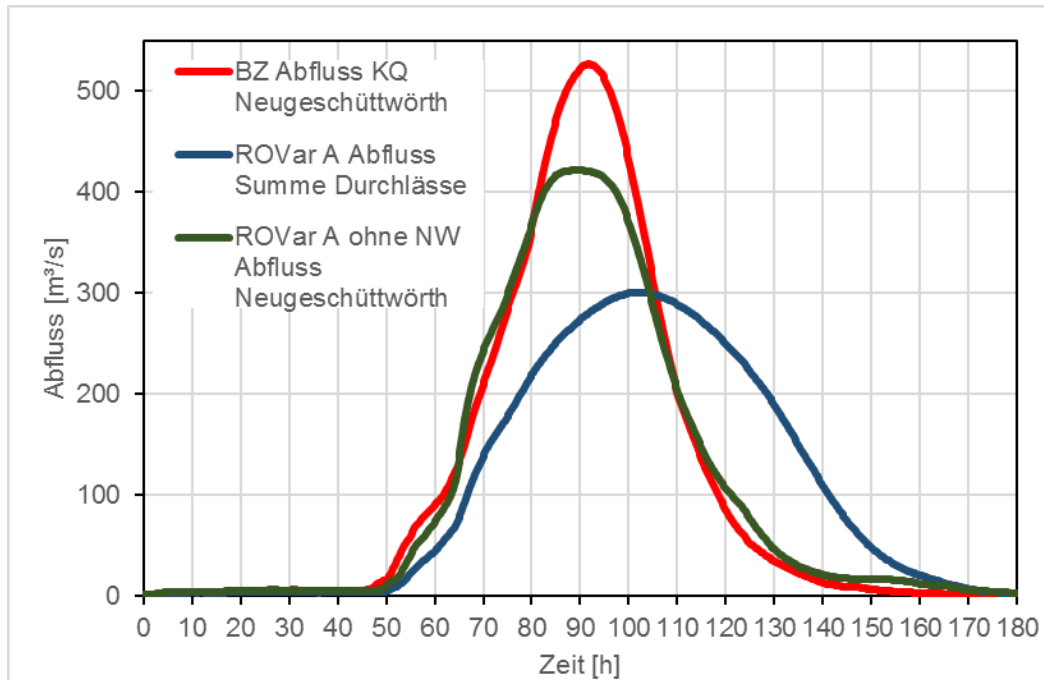
Abbildung 63: Neugeschüttwörth, ROVar A ohne Neugeschüttwörth (NW) - HQ_{\text{extrem}} , Ganglinie Kontrollquerschnitt (KQ) bzw. Auslassbauwerke
