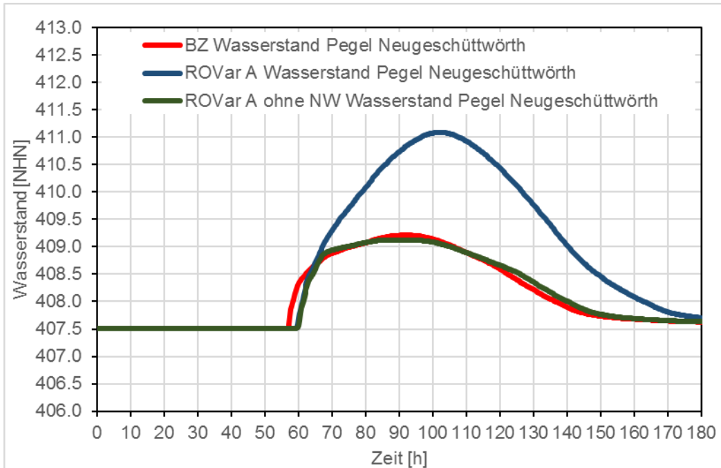
Abbildung 64: Neugeschüttwörth, ROVar A ohne Neugeschüttwörth - HQ_{\text{extrem}} , Pegelganglinie Kontrollquerschnitt bzw. Auslassbauwerke
