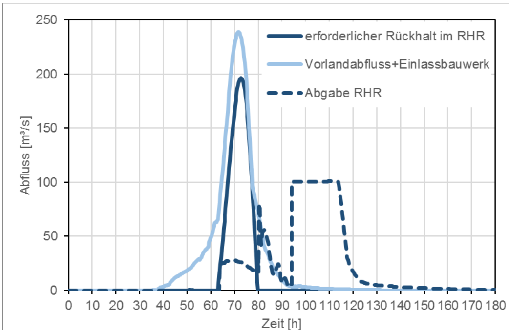
Abbildung 5: ROVar A HQ extrem , Erforderlicher Rückhalt im Rückhalteraum Leipheim, Zufluss und Abfluss des Rückhalterumes
