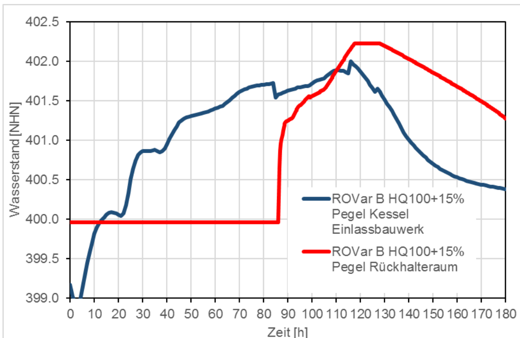
Abbildung 58: Donauwörth ROVar B - Projektteilziel 2, Pegelganglinien
