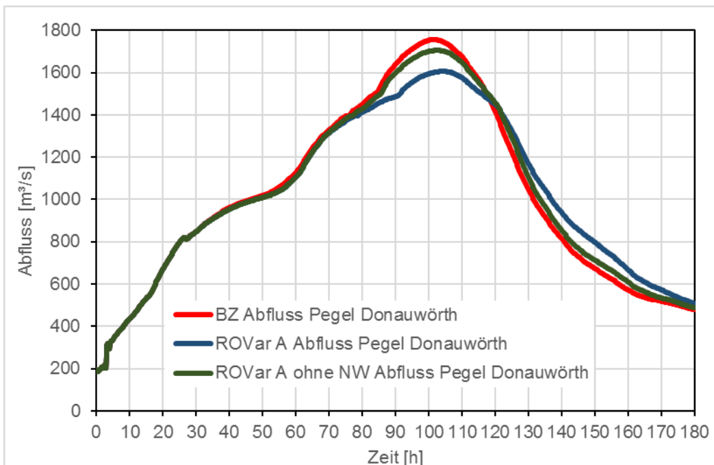
Abbildung 65: Pegel DON, ROVar A ohne Neugeschüttwörth - HQ_{\text{extrem}} , Abflussganglinien
