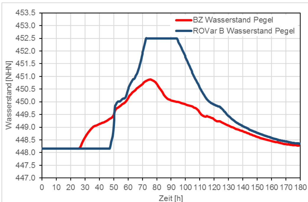
Abbildung 46: Leipheim ROVar B - Projektteilziel 1, Pegelganglinien
