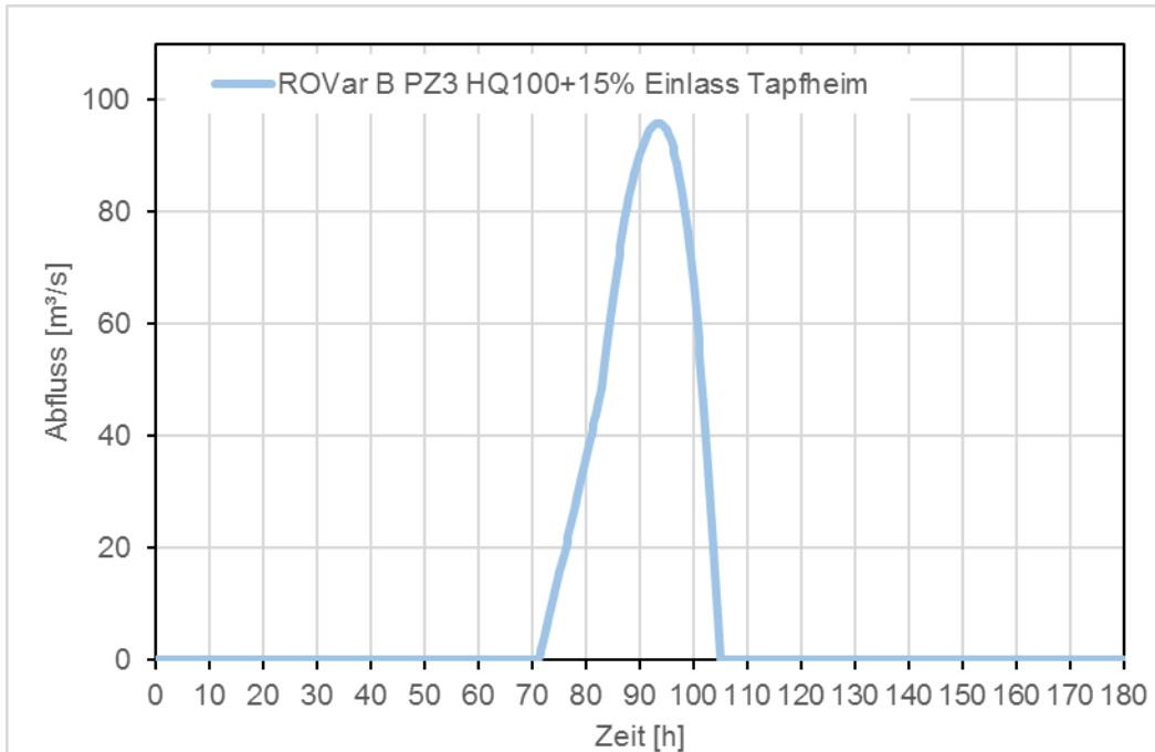
Abbildung 22: ROVar B, Zufluss in den Rückhalteraum Tapfheim zur Scheitelkappung
