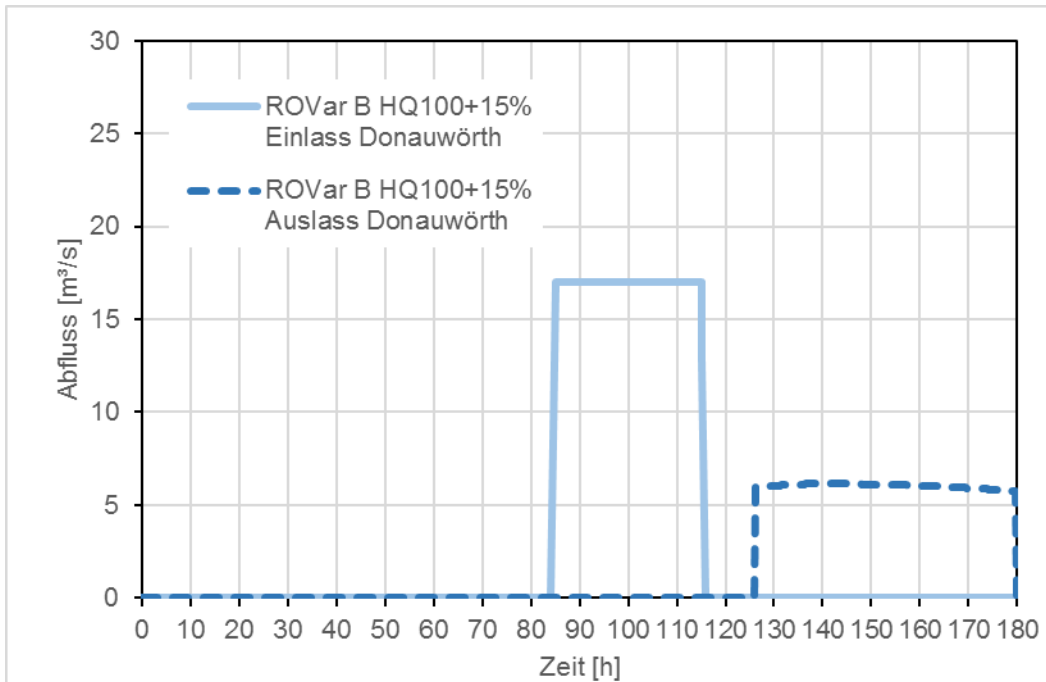
Abbildung 57: Donauwörth ROVar B - Projektteilziel 2, Ganglinien Ein- und Auslassbauwerke
