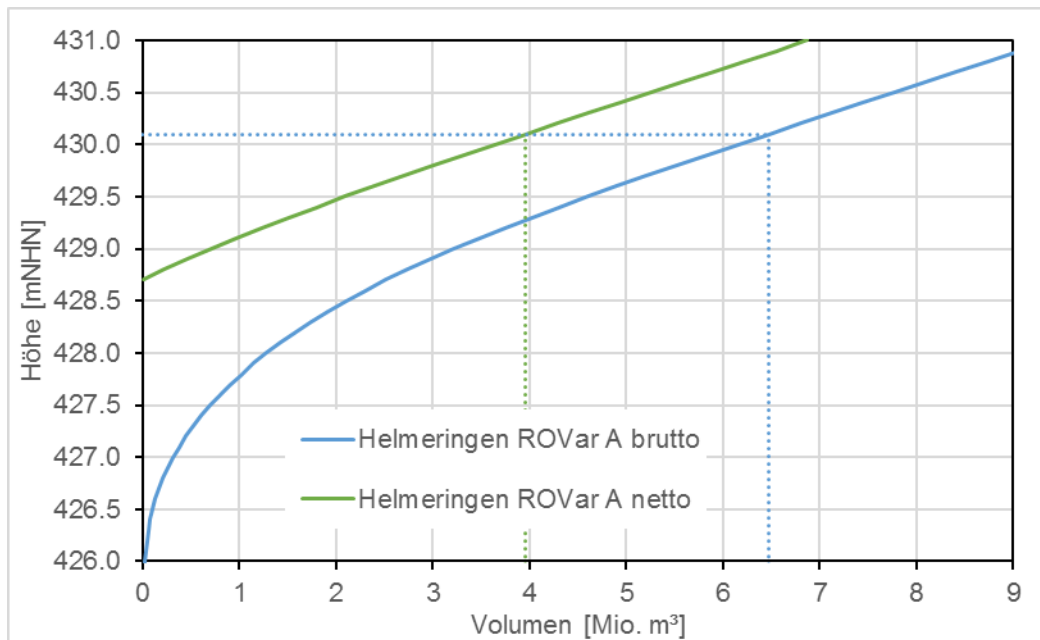
Abbildung 8: Speicherinhaltslinie Rückhalteraum Helmeringen
