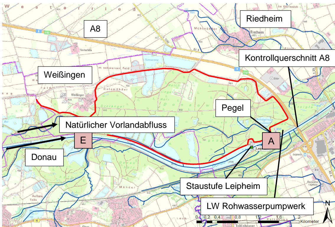
Abbildung 1: Rückhalteraum Leipheim, ROVar A, (E = Einlassbauwerk, A = Auslassbauwerk)
