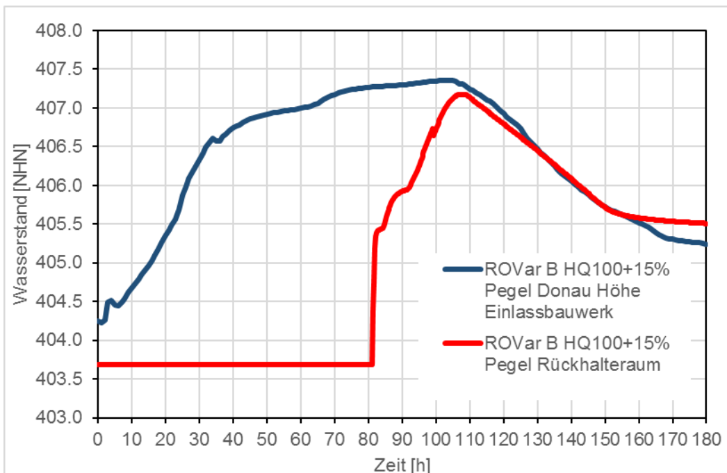
Abbildung 56: Tapfheim ROVar B - Projektteilziel 2, Pegelganglinien
