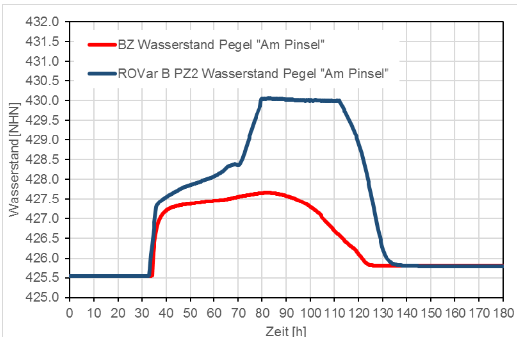
Abbildung 49: Helmeringen ROVar B - Projektteilziel 1, Pegelganglinien
