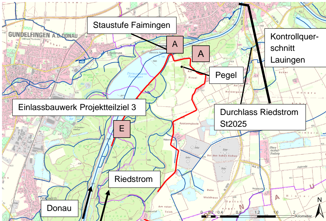
Abbildung 6: Rückhalteraum Helmeringen, ROVar A
