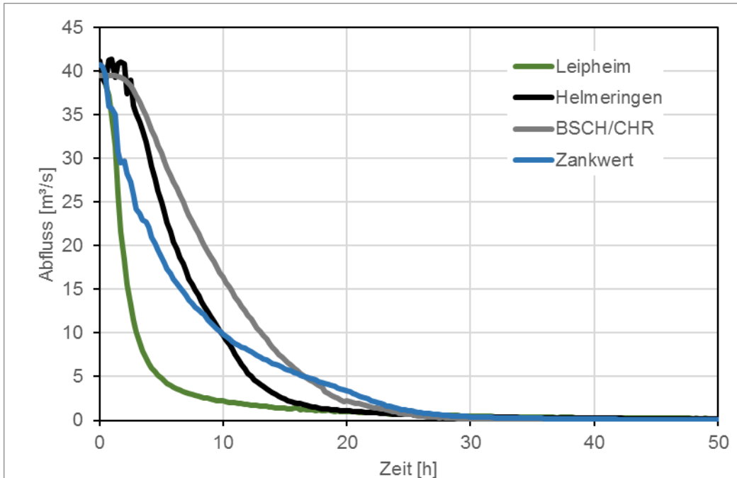
Abbildung 62: Ökologische Flutungen Abfluss am Auslass, Leerungsvorgang
