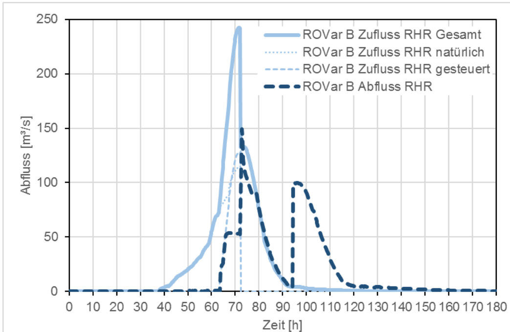
Abbildung 45: Leipheim ROVar B - Projektteilziel 1, Ganglinien Ein- und Auslassbauwerke
