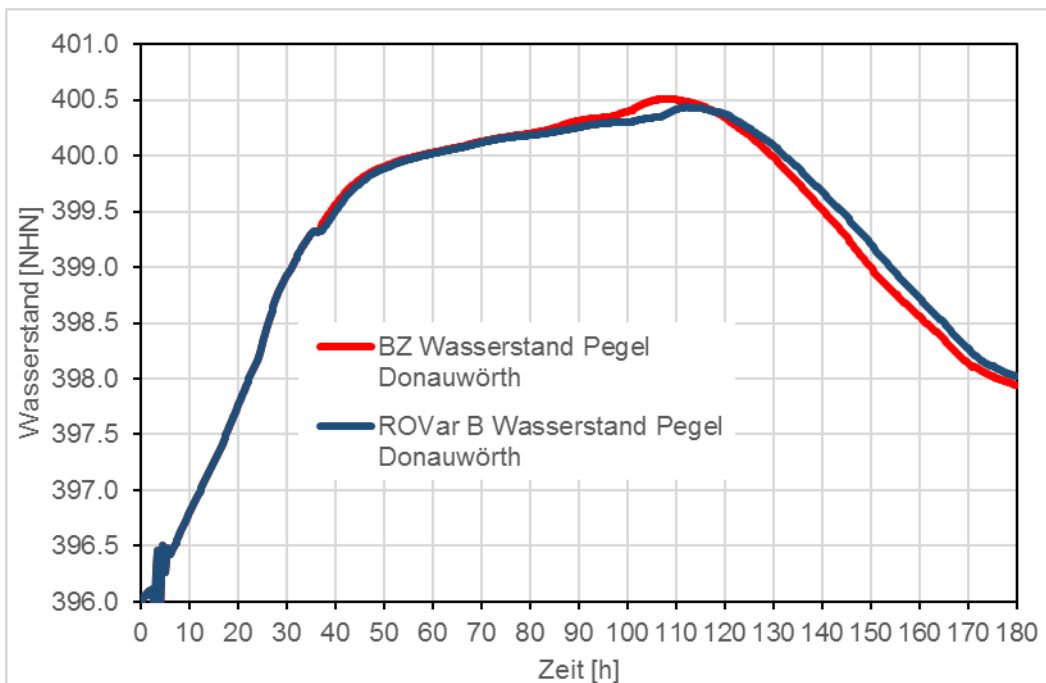
Abbildung 60: Pegel DON, ROVar B - Projektteilziel 2, Pegelganglinien
