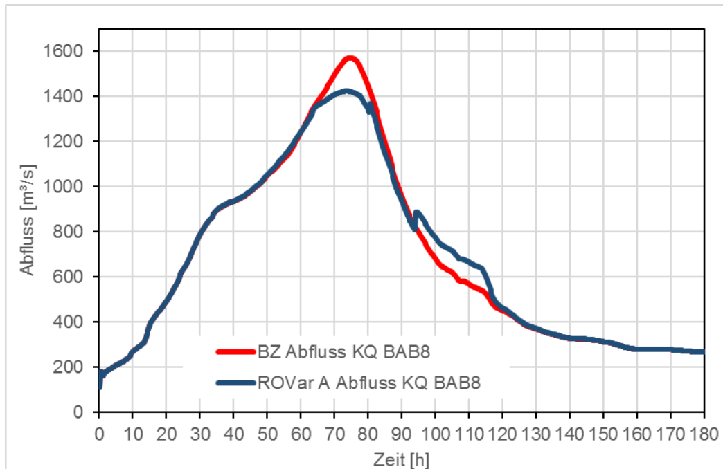
Abbildung 30: Leipheim ROVar A - Projektteilziel 1, Abflussganglinien Kontrollquerschnitt BAB8
