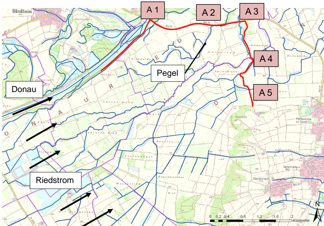
Abbildung 13: Rückhalteraum Neugeschüttwörth, ROVar A
