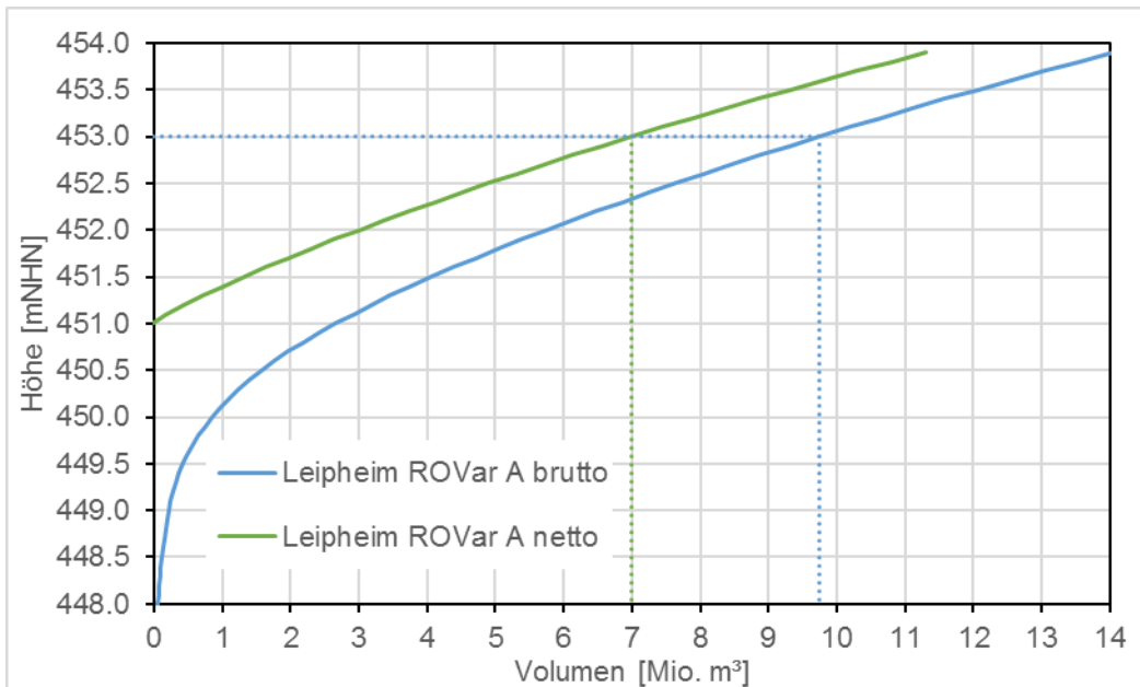
Abbildung 2: Speicherinhaltslinie Rückhalteraum Leipheim ROVar A
