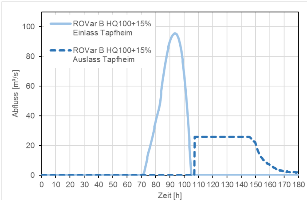
Abbildung 55: Tapfheim ROVar B - Projektteilziel 2, Ganglinien Ein- und Auslassbauwerke
