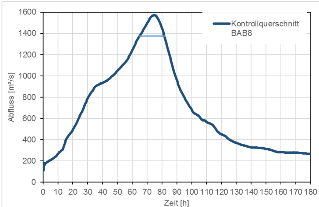
Abbildung 3: Bezugszustand HQ_{\text{extrem}} , Kontrollquerschnitt BAB8, Zielwert Scheitelkapung
