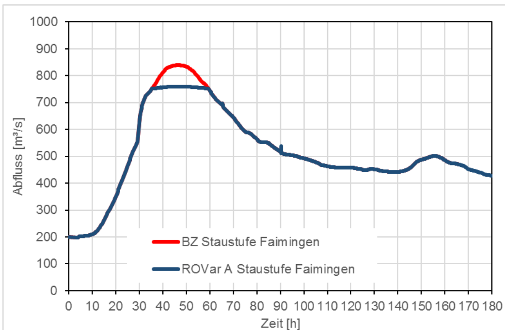
Abbildung 41: Helmeringen ROVar A - Projektteilziel 3, Abflussganglinien an der Staustufe Faimingen
