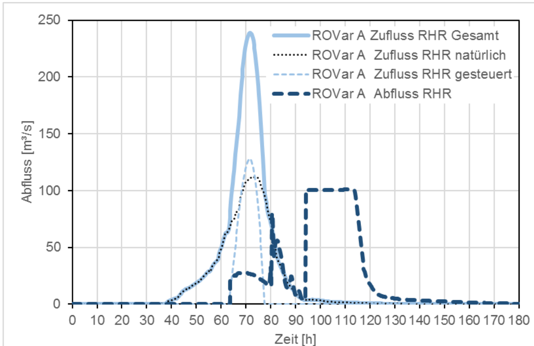
Abbildung 31: Leipheim ROVar A - Projektteilziel 1, Ganglinien Ein- und Auslassbauwerke
