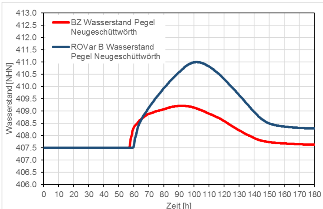
Abbildung 52: Neugeschüttwörth ROVar B - Projektteilziel 1, Pegelganglinien
