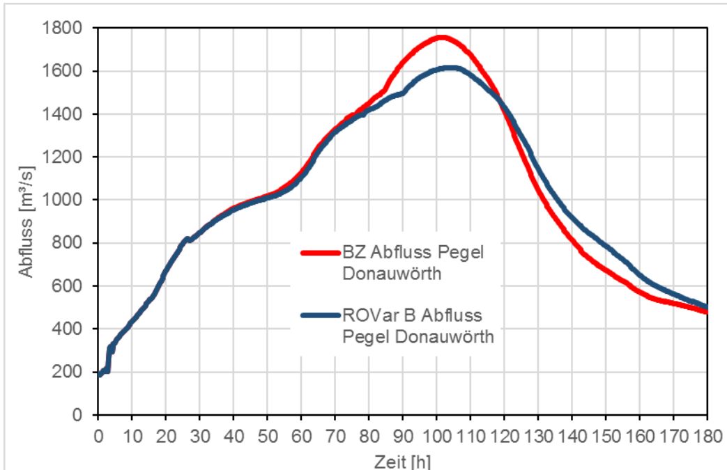
Abbildung 53: Pegel DON, ROVar B - Projektteilziel 1, Abflussganglinien
