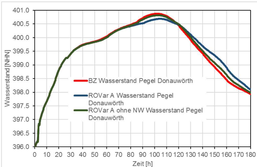
Abbildung 66: Pegel DON, ROVar A ohne Neugeschüttwörth - HQ extrem , Pegelganglinien
