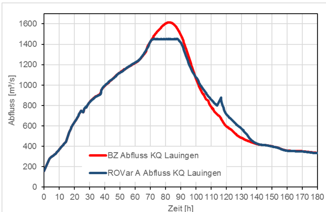
Abbildung 33: Helmeringen ROVar A - Projektteilziel 1, Abflussganglinien Kontrollquerschnitt Lauingen
