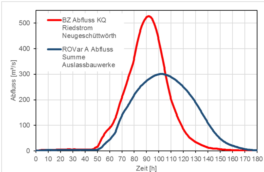
Abbildung 36: Neugeschüttwörth ROVar A - Projektteilziel 1, Ganglinie Kontrollquerschnitt im Riedstrom bzw. Durchlassbauwerke
