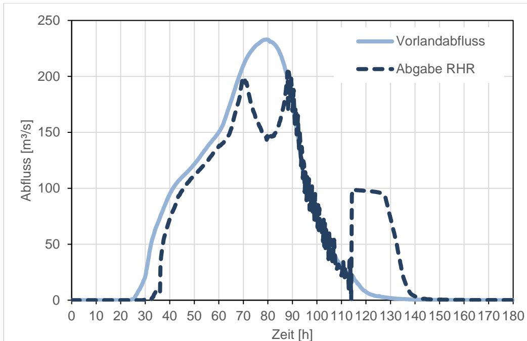
Abbildung 10: ROVar A, Zufluss in den Rückhalteraum Helmeringen und Abfluss entsprechend der benötigten Scheitelkappung
