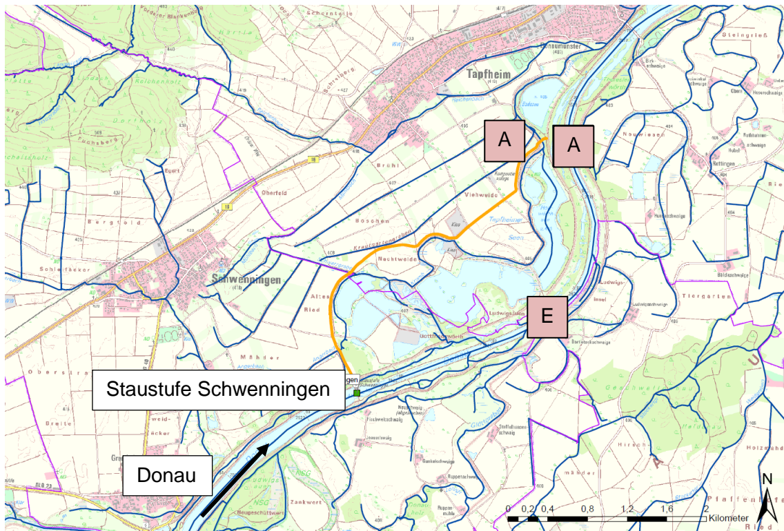
Abbildung 21: Rückhalteraum Tapfheim, ROVar B
