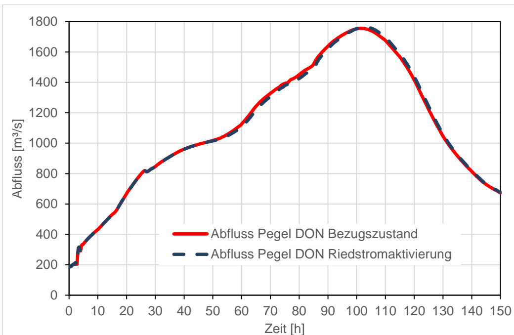
Abbildung 68: Abflussganglinien am Pegel Donauwörth im Bezugzustand und im Fall der Riedstromaktivierung
