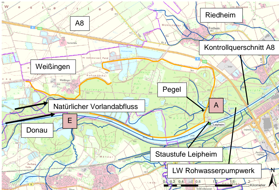
Abbildung 15: Rückhalteraum Leipheim, ROVar B
