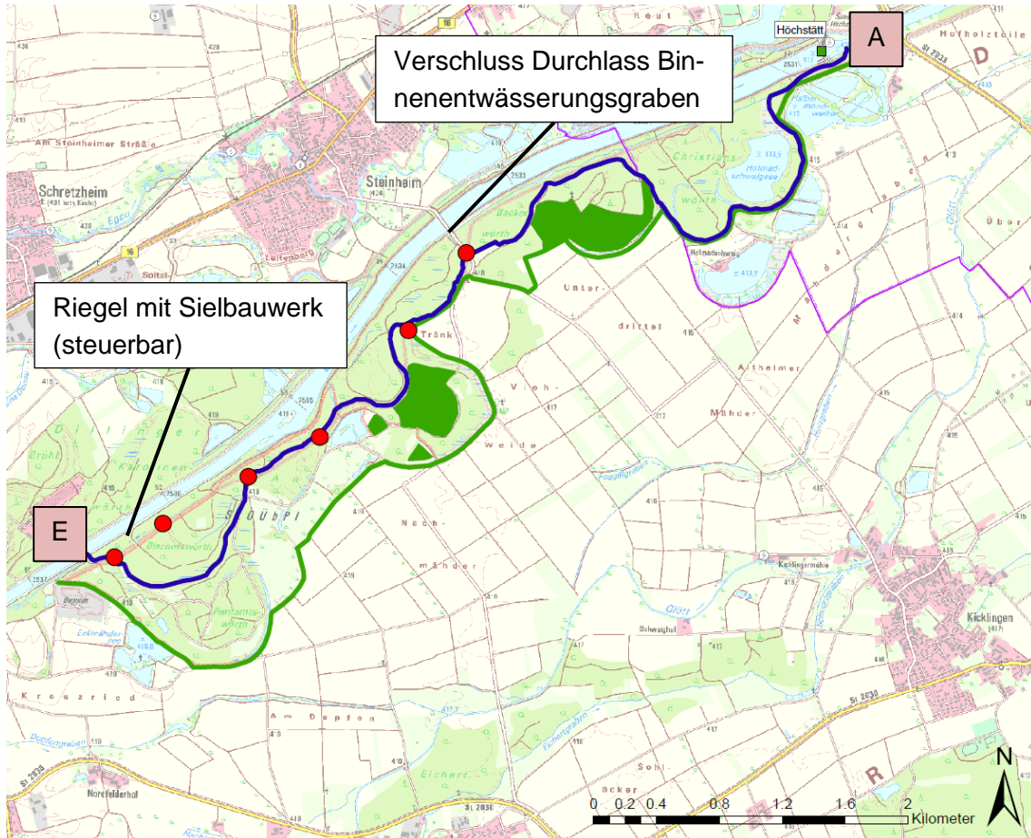
Abbildung 27: Bischofswörth/Christianswörth, Gerinne für ökologische Flutungen (blau), Deichrückbau (rot), „disable“-Elemente grün
