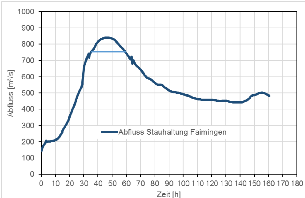
Abbildung 11: Bezugszustand HQ1994 angepasst, Kontrollquerschnitt Stauhaltung Faimingen, Zielwert Scheitelkappung
