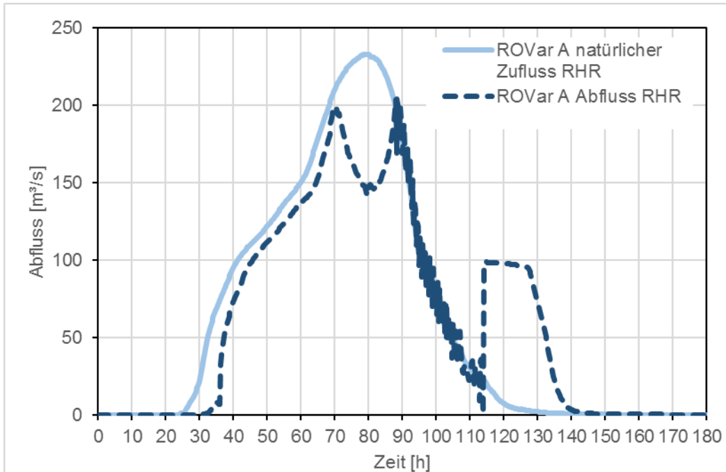
Abbildung 34: Helmeringen ROVar A - Projektteilziel 1, Ganglinien Ein- und Auslassbauwerke
