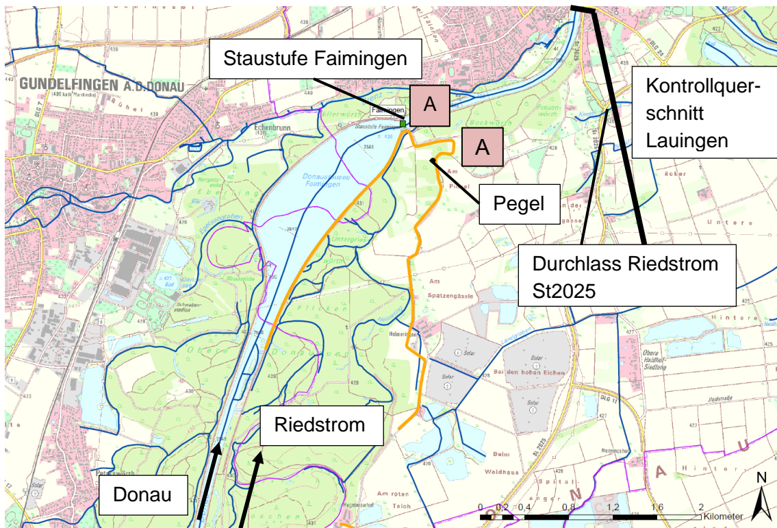
Abbildung 17: Rückhalteraum Helmeringen, ROVar B
