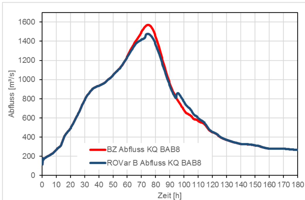
Abbildung 44: Leipheim ROVar B - Projektteilziel 1, Abflussganglinien Kontrollquerschnitt BAB8
