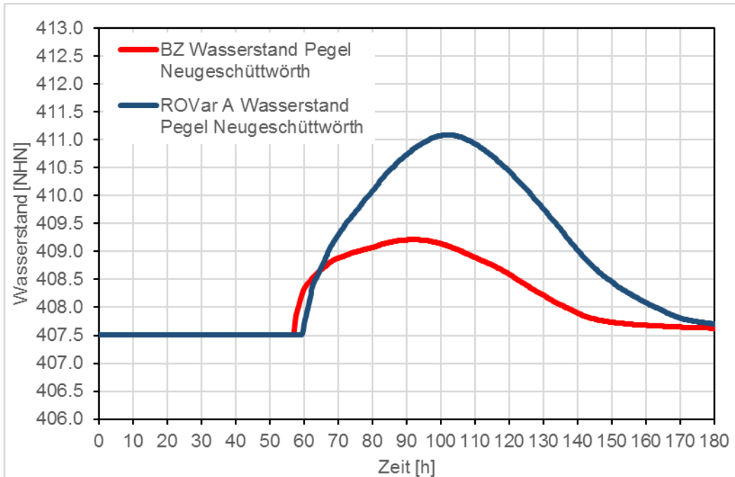
Abbildung 38: Neugeschüttwörth ROVar A - Projektteilziel 1, Wasserstandsganglinien im Rückhalteraum
