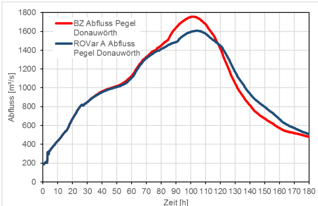
Abbildung 39: Pegel DON, ROVar A - Projektteilziel 1, Abflussganglinien
