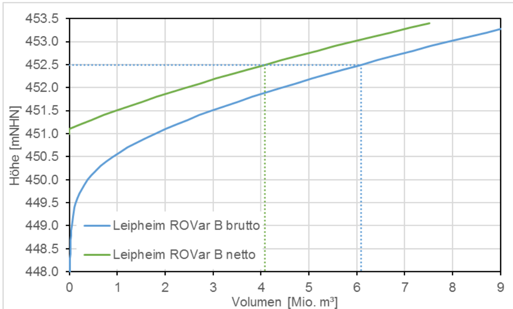
Abbildung 16: Speicherinhaltslinie Rückhalteraum Leipheim ROVar B
