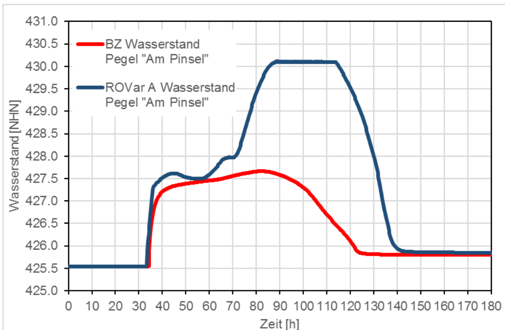
Abbildung 35: Helmeringen ROVar A - Projektteilziel 1, Wasserstandsganglinien im Rückhalteraum
