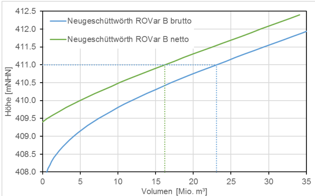
Abbildung 20: Speicherinhaltslinie Rückhalteraum Neugeschüttwörth ROVar B
