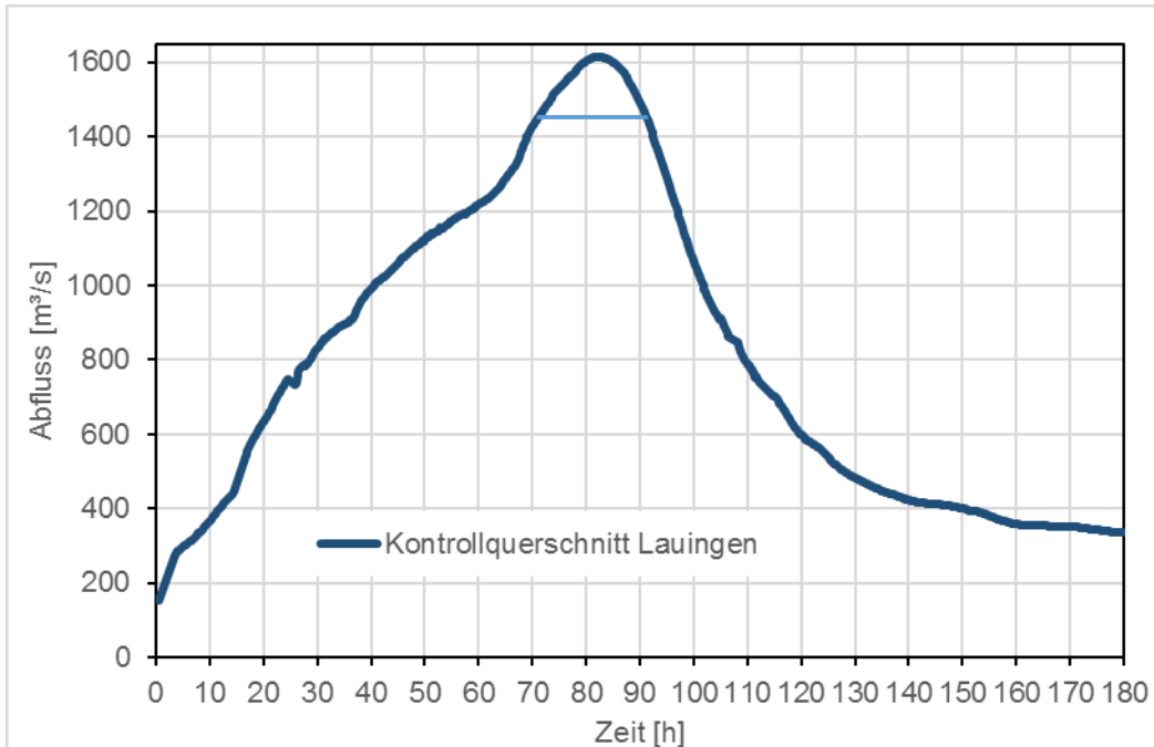
Abbildung 9: Bezugszustand HQ_{\text{extrem}} , Kontrollquerschnitt Lauingen, Zielwert Scheitelkappung
