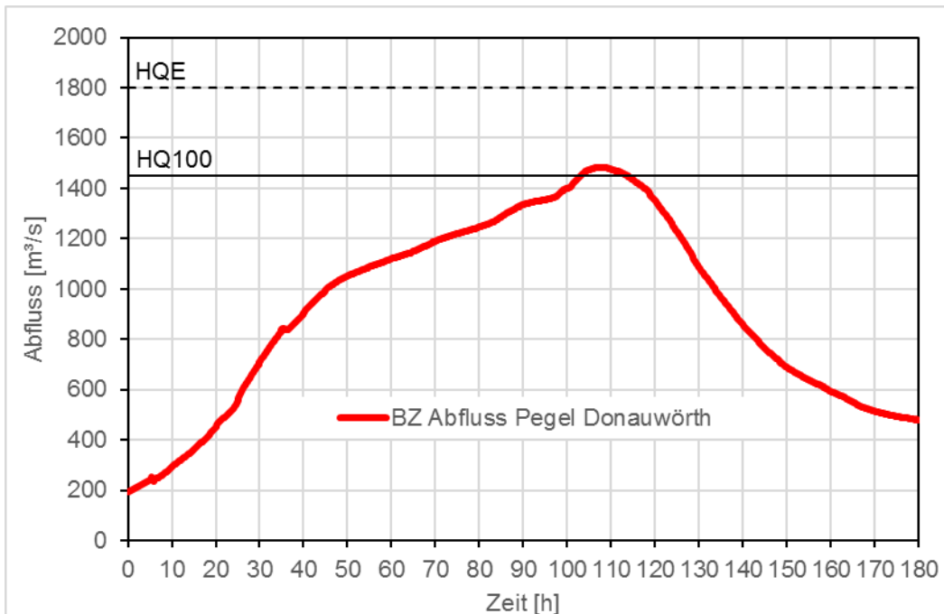
Abbildung 29: Bezugszustand, HQ 100 zzgl. Klimafaktor: Abflussganglinie am Pegel Donauwörth
