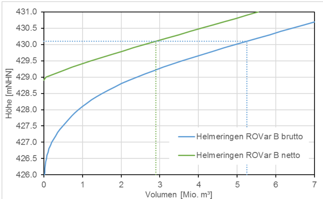
Abbildung 18: Speicherinhaltslinie Rückhalteraum Helmeringen ROVar B
