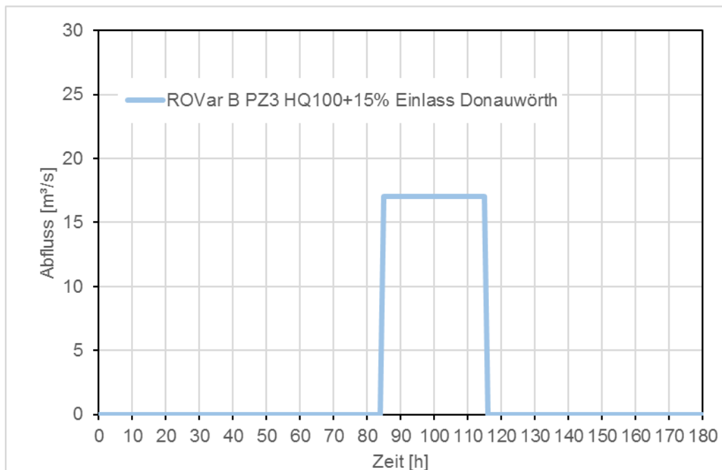
Abbildung 24: ROVar B, Zufluss in den Rückhalterraum Donauwörth
