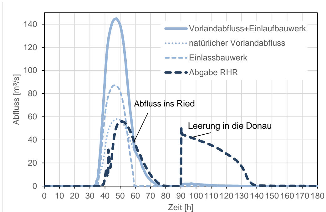
Abbildung 12: ROVar A HQ1994 angepasst, Zu- und Abfluss des Rückhalteraumes Helmeringen
