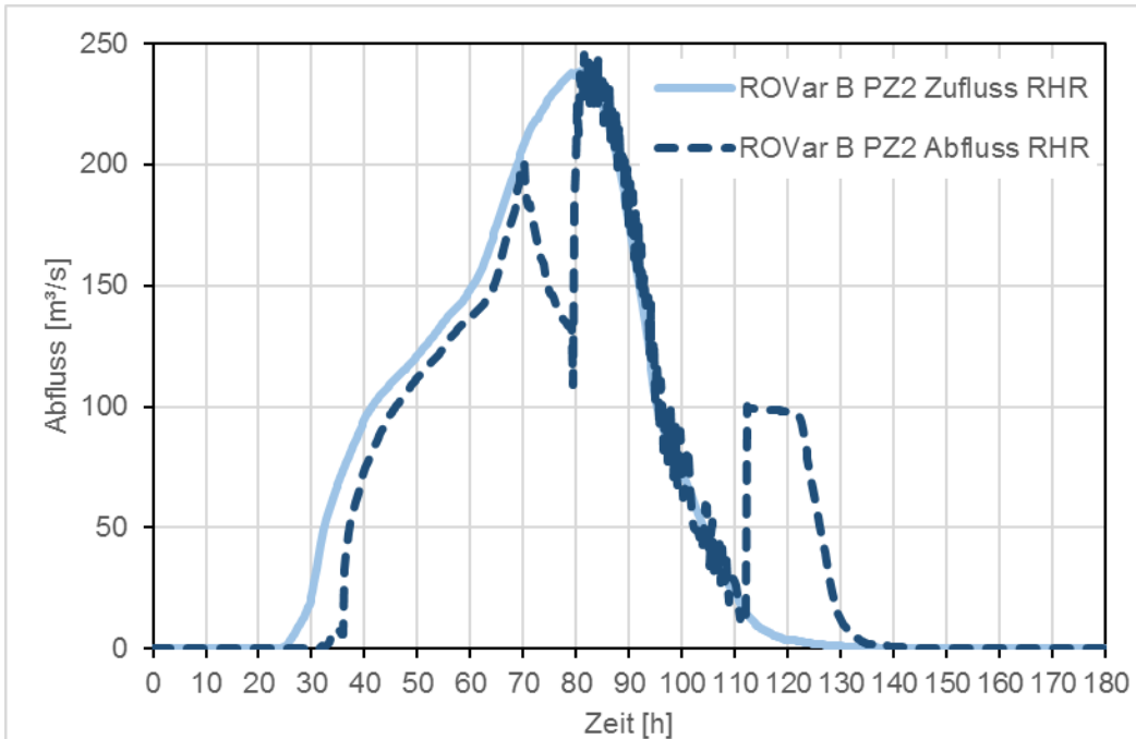
Abbildung 48: Helmeringen ROVar B - Projektteilziel 1, Ganglinien Ein- und Auslassbauwerke
