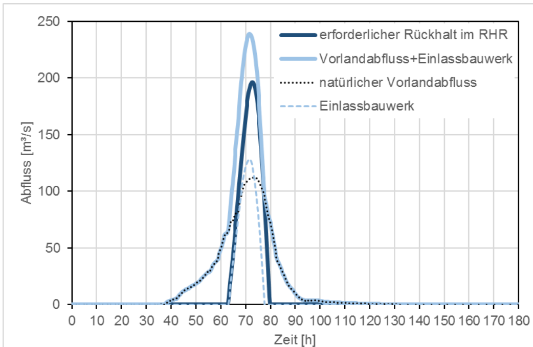
Abbildung 4: ROVar A, Zuflüsse in den Rückhalteraum Leipheim und erforderlicher Rückhalt zur Scheitelkappung
