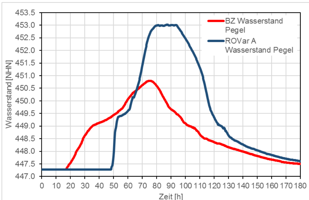
Abbildung 32: Leipheim ROVar A - Projektteilziel 1, Wasserstandsganglinien im Rückhalteraum
